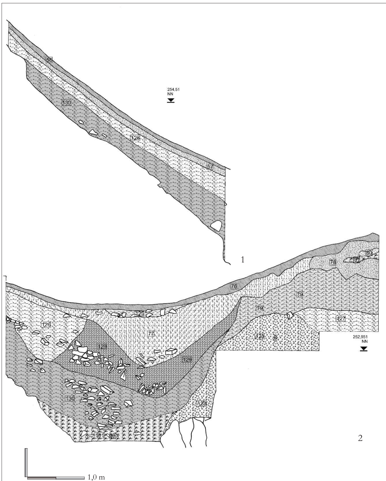
Tafel 20 Haibach, Ketzelsburg 1: Schnitt XV, Profil 2; 2: Schnitt XIV, Profil 4. M. 1 : 40.
